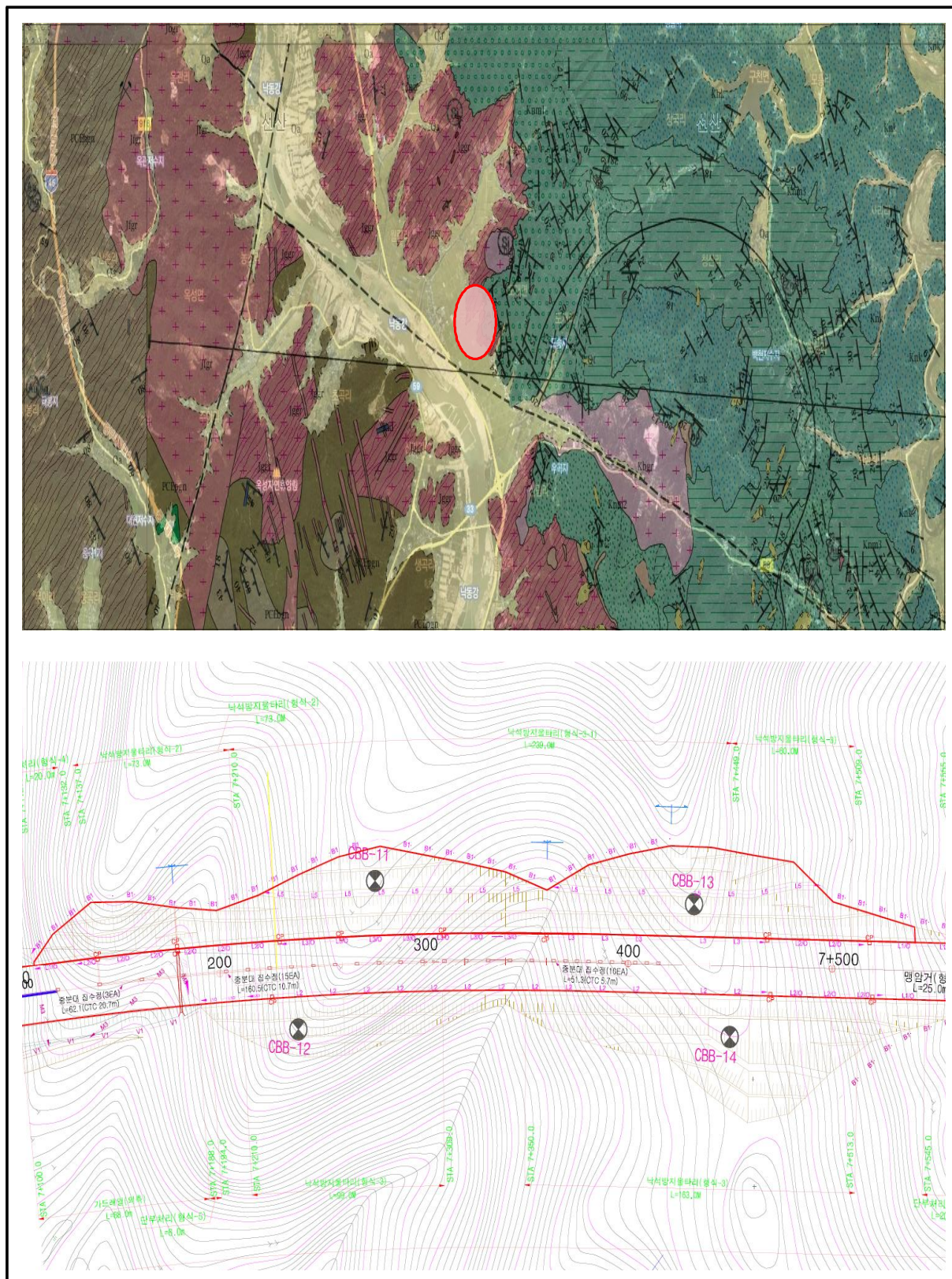
【그림 9.14】 상주절토09 검토대상 비탈면구간
