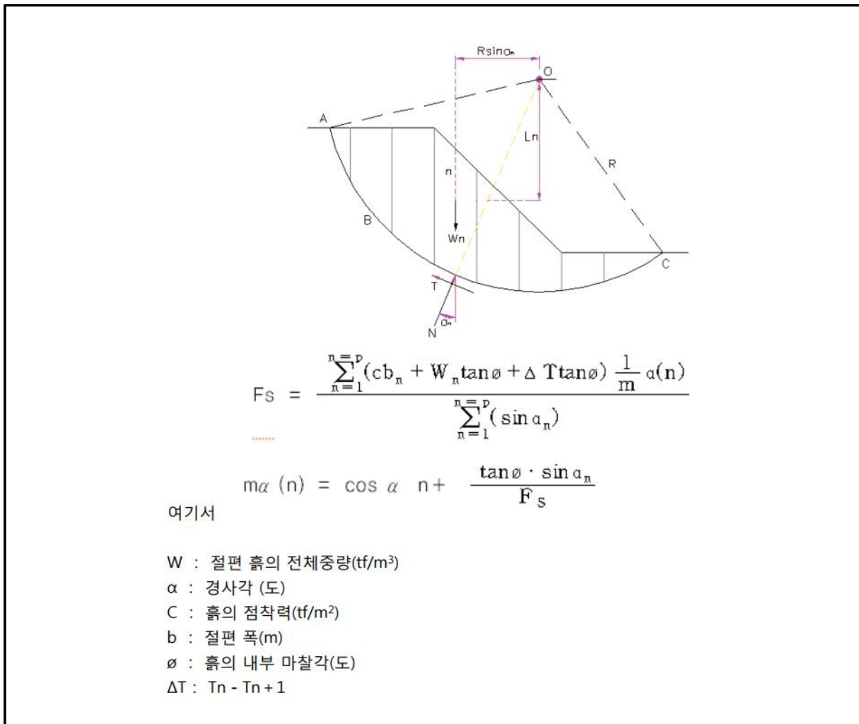
【그림 9.7】 Bishop의 안전율 계산식
