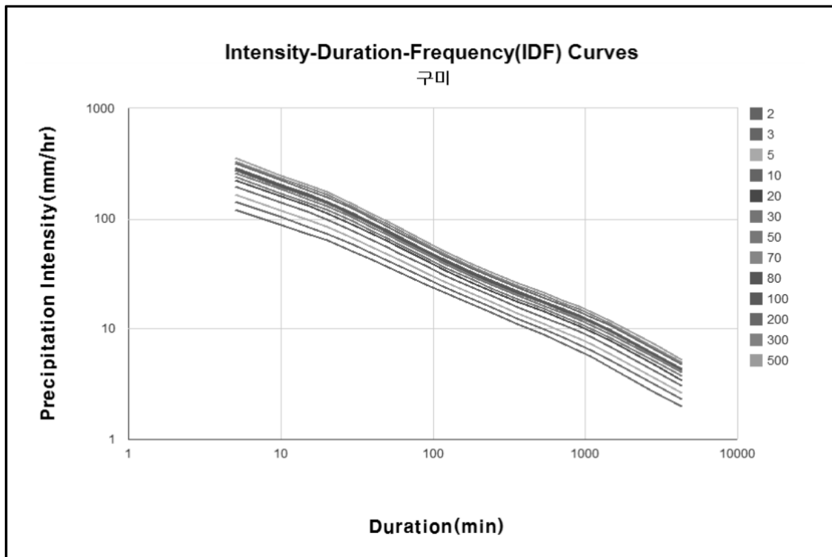
【그림 9.9】 구미지역 IDF곡선
